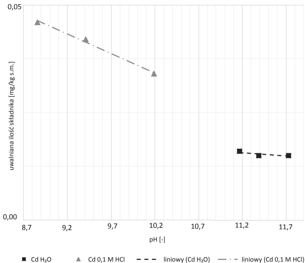
Ryc. 4. Uwalnianie kadmu z z c wiesiny tw. rdniejącej w zależności od cieczy wmywającej i pH eluatu
